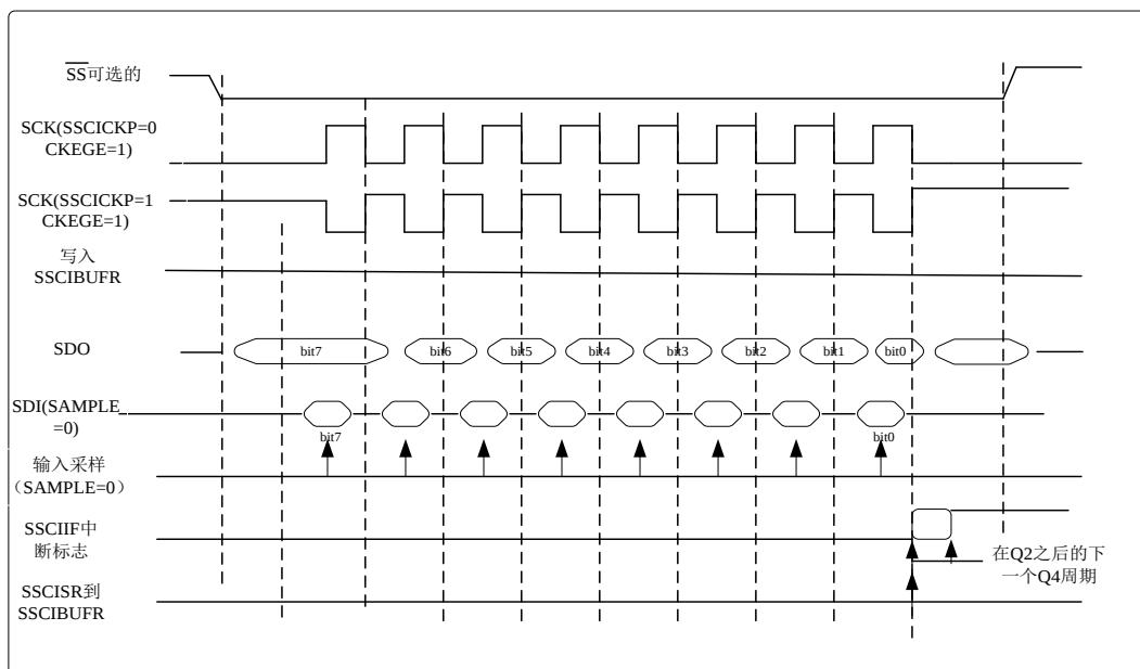
图 0.33 SPI 模式时序图（从动模式且 CKEGE=1）
