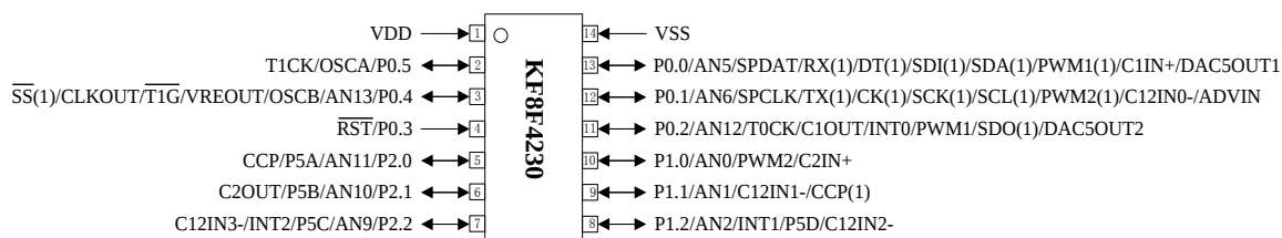
14 引脚示意图:
