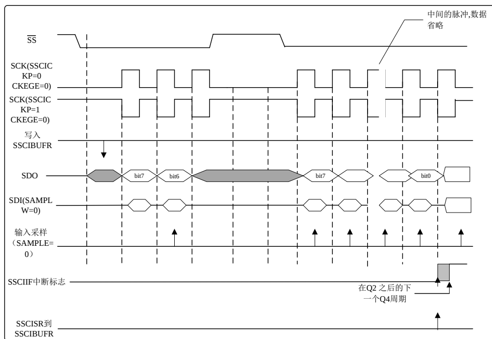
图 0.31 从动时序图
