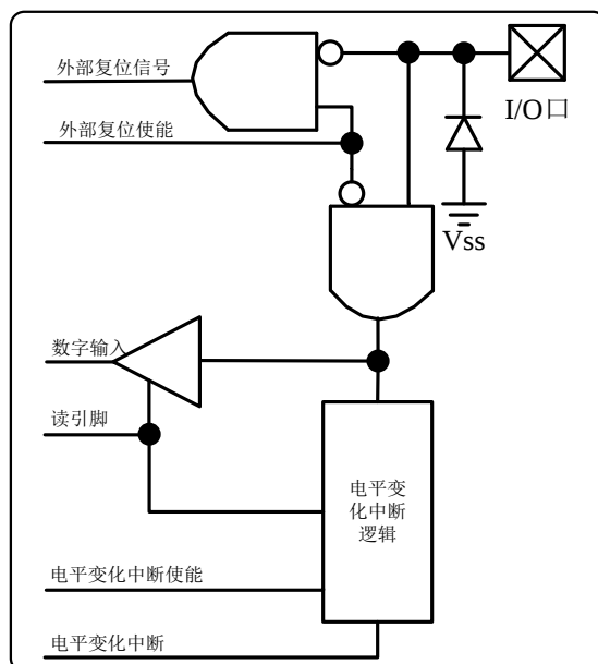
图 2.2 引脚 P0.3 原理功能框图
