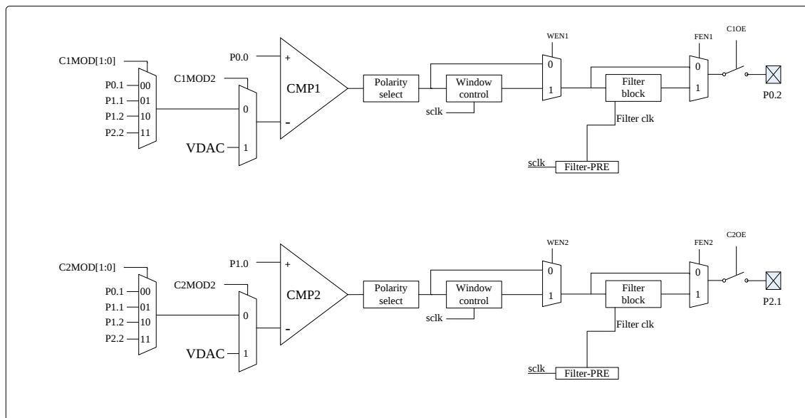
图 0.1 模拟比较器原理框图
