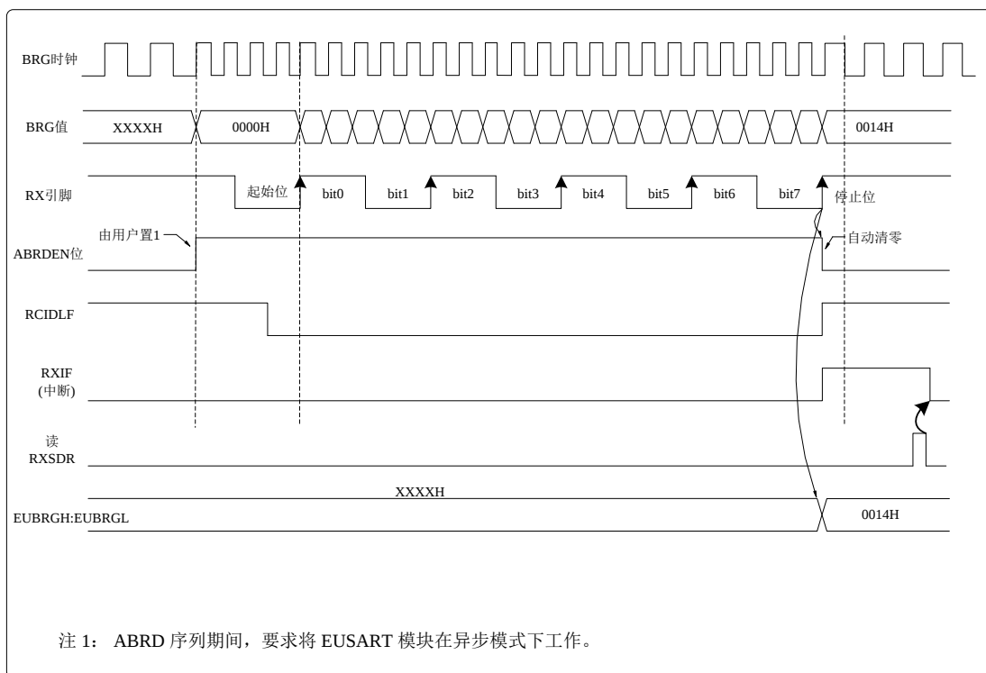
图 0.3 自动波特率检测
