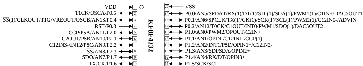
20 引脚示意图:
