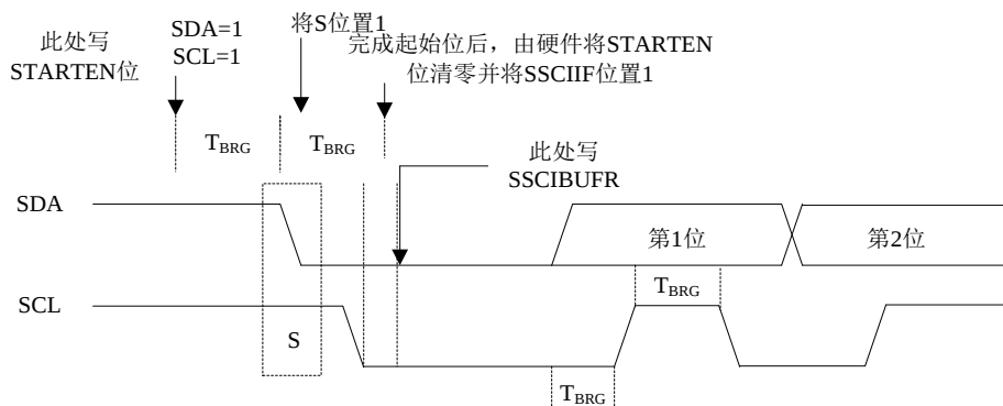
图 0.10 第一个启动位时序
