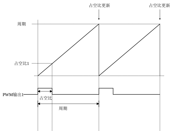
图 0.5 边沿对齐 PWM
