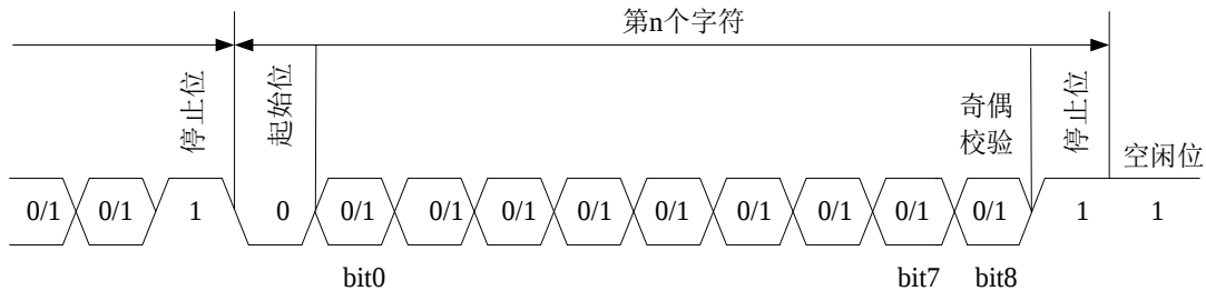
图 0.7 全双工异步通信数据结构图
