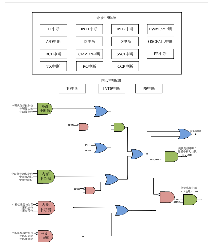
图 5.2 中断逻辑
