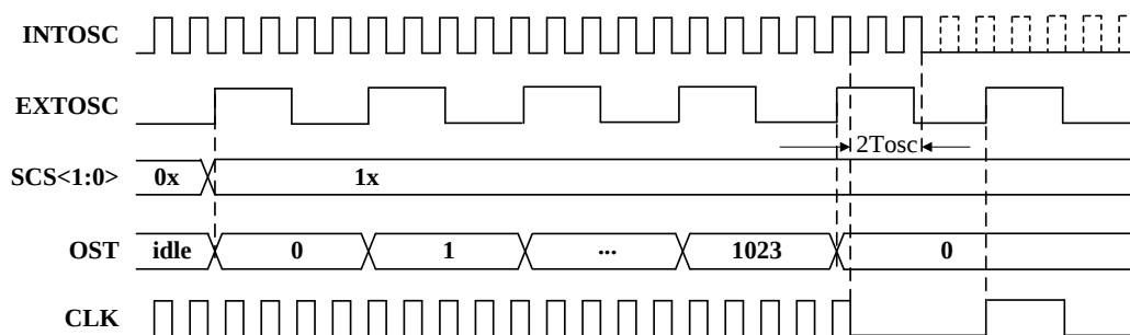
图 0.8 切换至外部时钟源时时钟信号同步时序图
