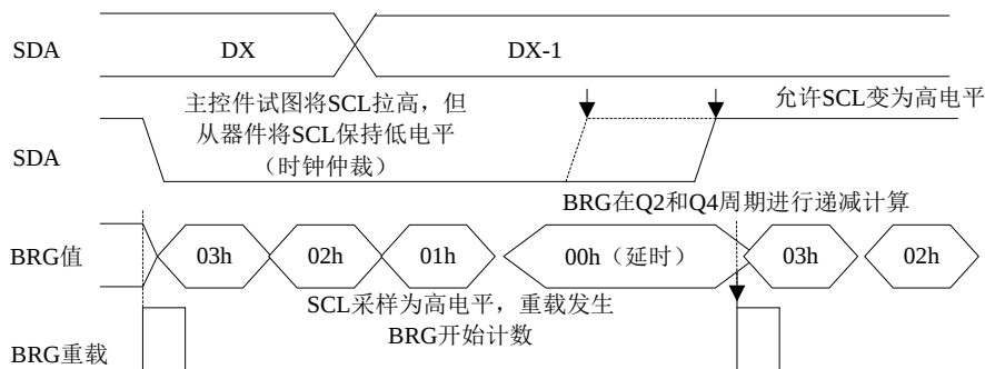
图 0.9 带有时钟仲裁的波特率发生器时序
