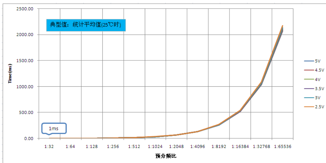
图 0.6 不同 VDD 时看门狗预分频比 一周关系曲线图
