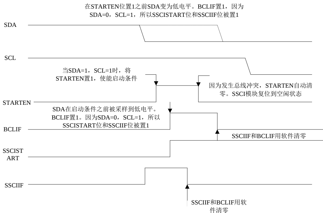
图 0.21 启动条件期间的总线冲突（仅 SDA）
