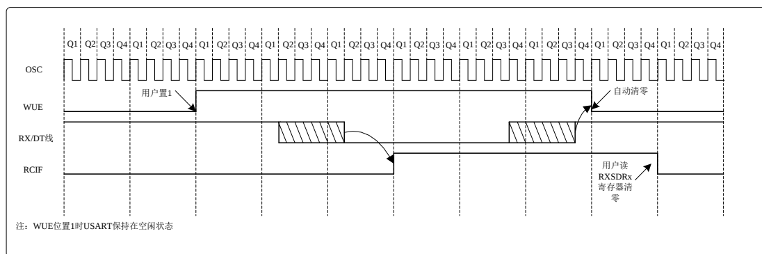
图 0.4 正常工作下的自动唤醒时序
