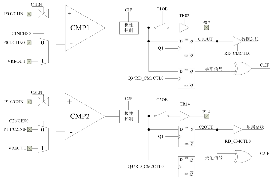
图 9.1 模拟比较器原理框图
