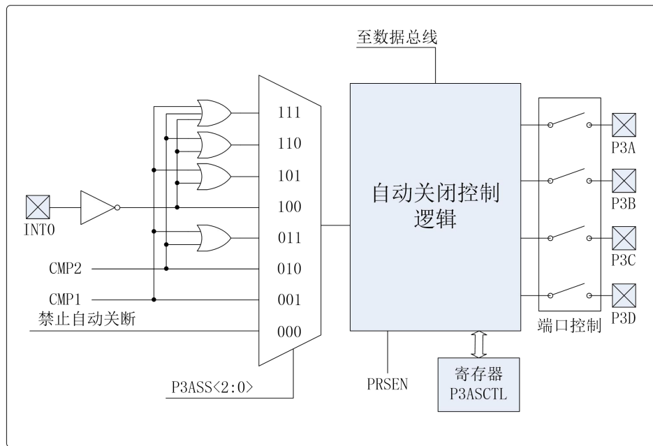
图 8.14 自动关断模式原理框图
