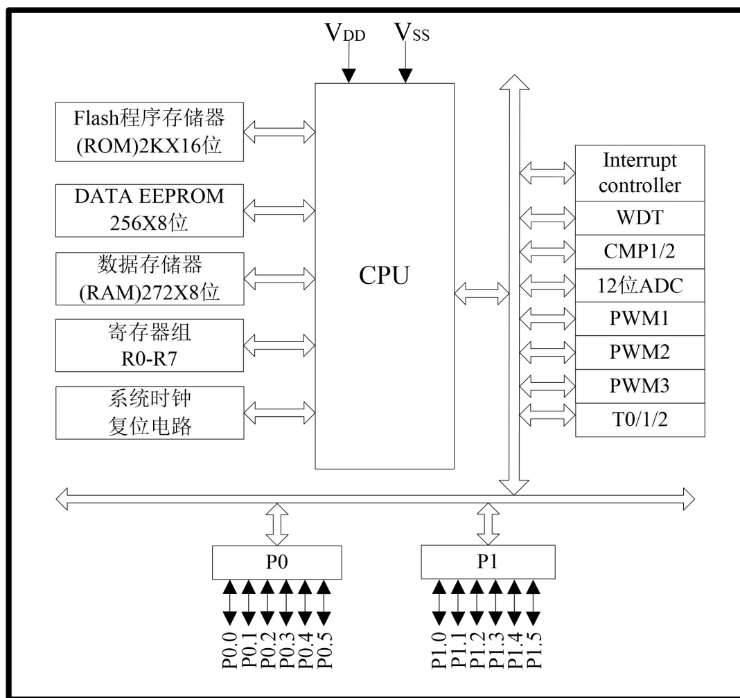
图 1.1: KF8F2320 系统框图
