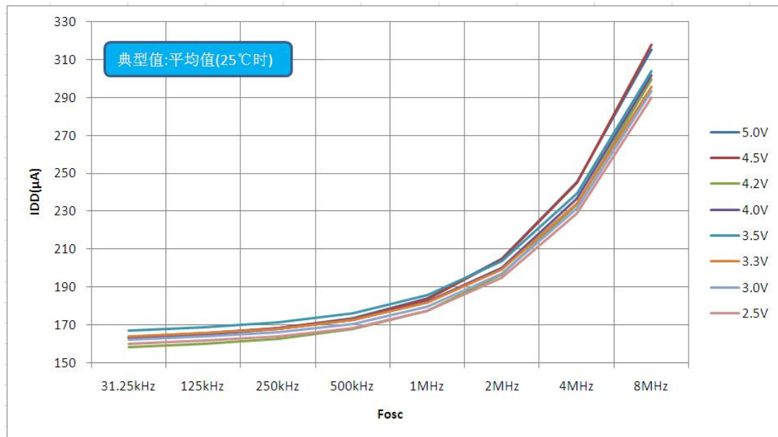
图 14 -1：不同 VDD 时典型 I_{DD} — F_{OSC} 关系曲线图
