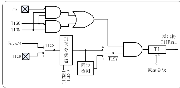
图 6.2 T1 原理框图
