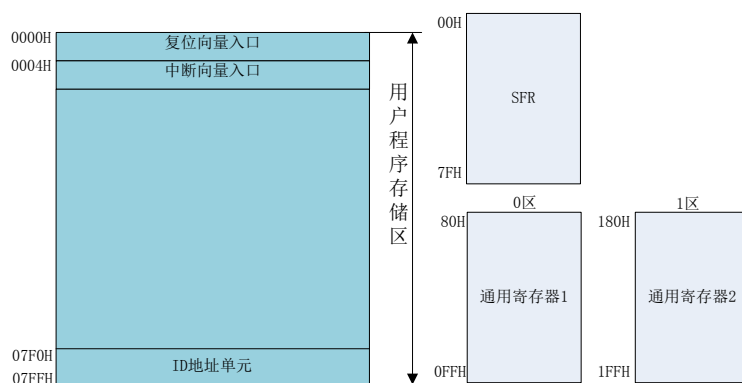
图 3.1 KF8F2320 存储器组织图
