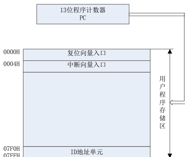
图 3.3 KF8F2320 程序存储器映射
