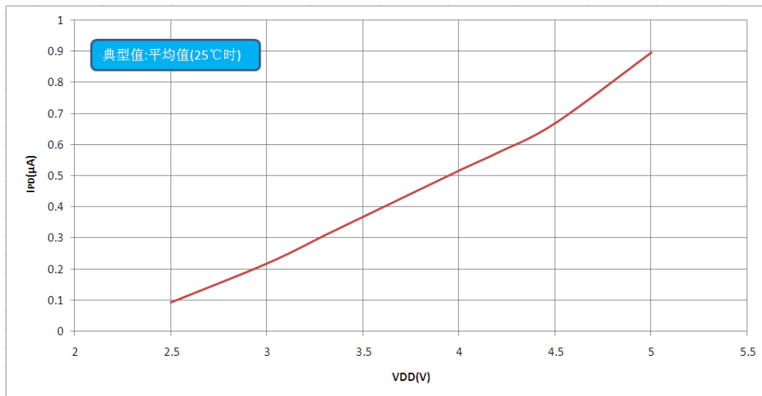
图 14-2：不同 VDD 时典型 I PD — VDD 关系曲线图
