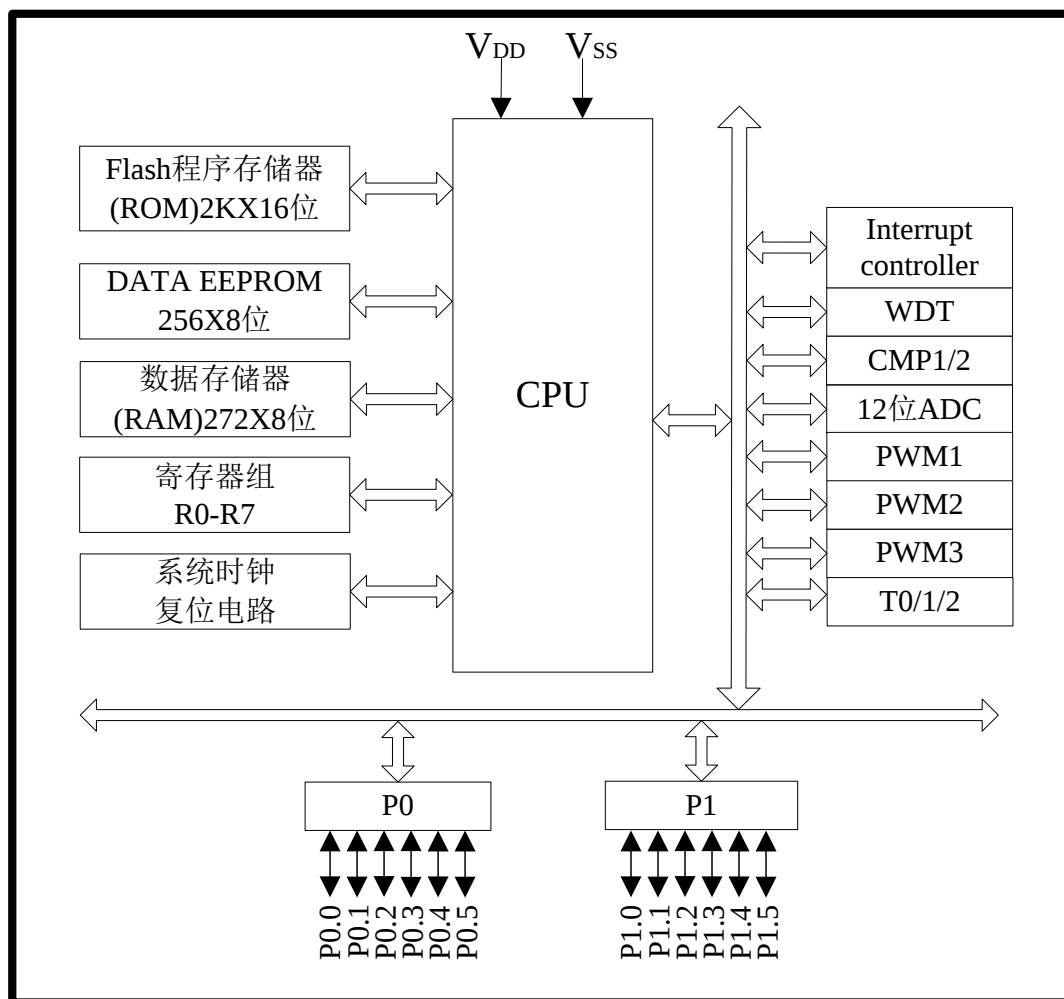
图 1.1: KF8F2320 系统框图
