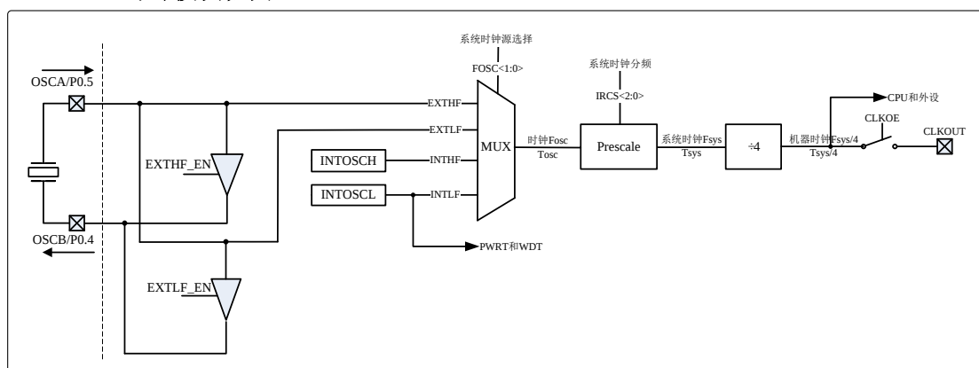
图 1.3 时钟模块框图
