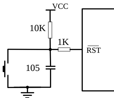
图 11.2 建议 \overline{RST} 复位电路
