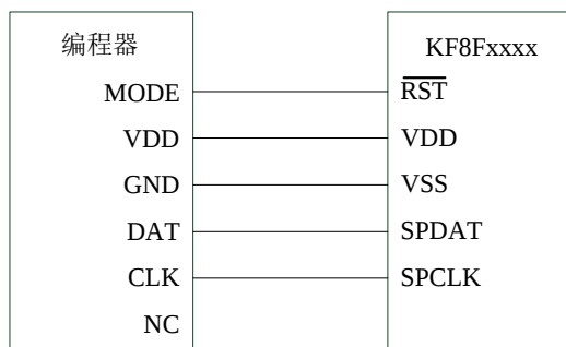
图 1.5 KF8F2320 在线串行编程连接图
