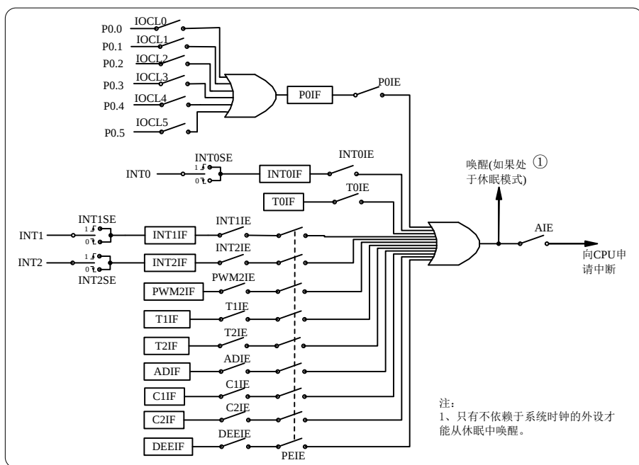
图 5.1 中断逻辑
