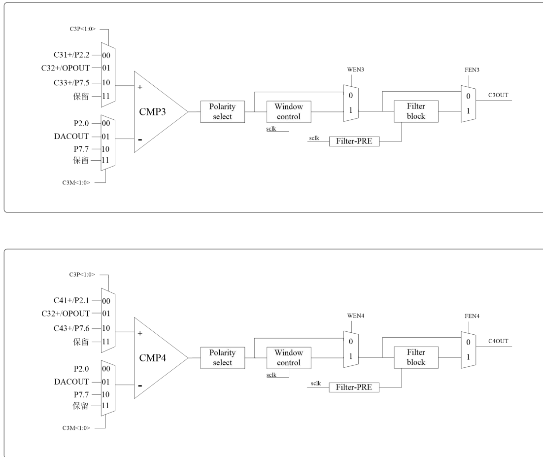
图 12.1 模拟比较器模块框图
