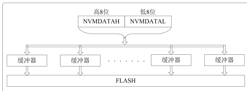
图 3.8 写操作
