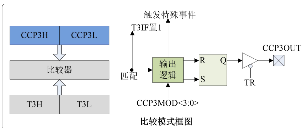
图6.6 比较模式原理框图
