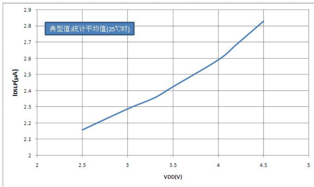
图25.3: 不同VDD 时典型IDSLP — VDD 关系曲线图(深度休眠模式, 禁止所有外设)
