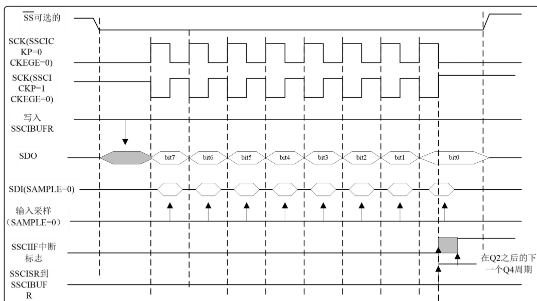
图13.32 SPI模式时序图（从动模式且CKEGE=0）
