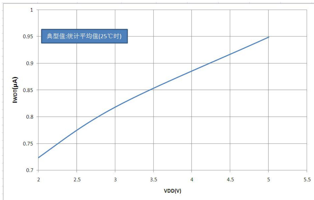
图25.7:看门狗电流 I_{WDT} — V_{DD} 关系曲线图
