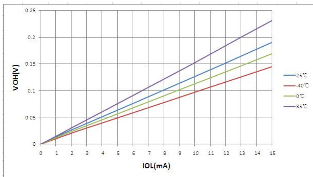
图25.17:不同温度时 V_{OH} — I_{OL} 关系曲线图 ( V_{DD} = 5.0V )
