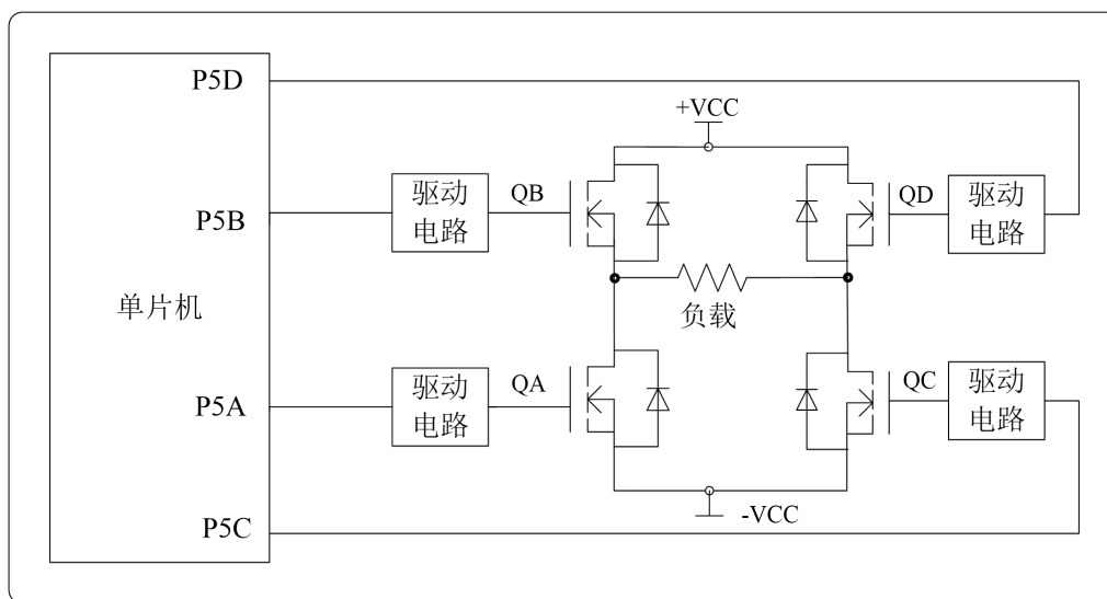
图 10.13 全桥输出模式应用电路示例
