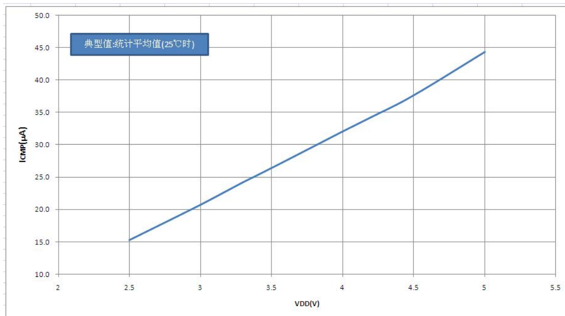
图25.8:比较器电流 I_{CMP} — V_{DD} 关系曲线图（使能一路比较器）
