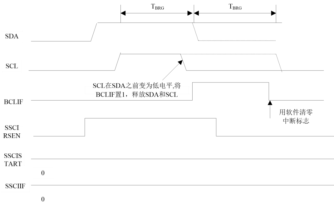
图 13.25 重复启动条件期间的总线冲突（情形 2）
