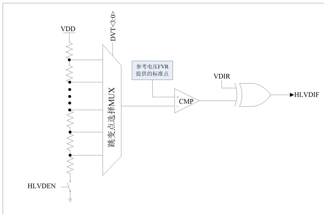
图：高低压检测原理图
