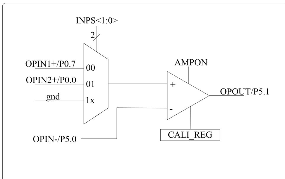
图 11.1 运放内部框图
