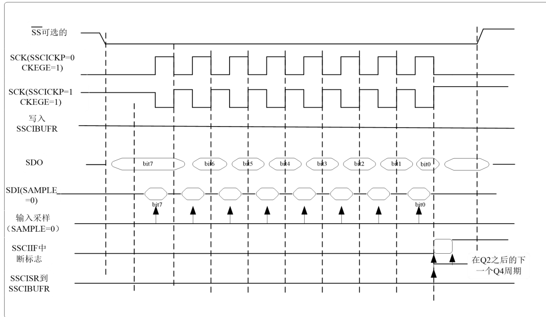
图 13.33 SPI 模式时序图（从动模式且 CKEGE=1）
