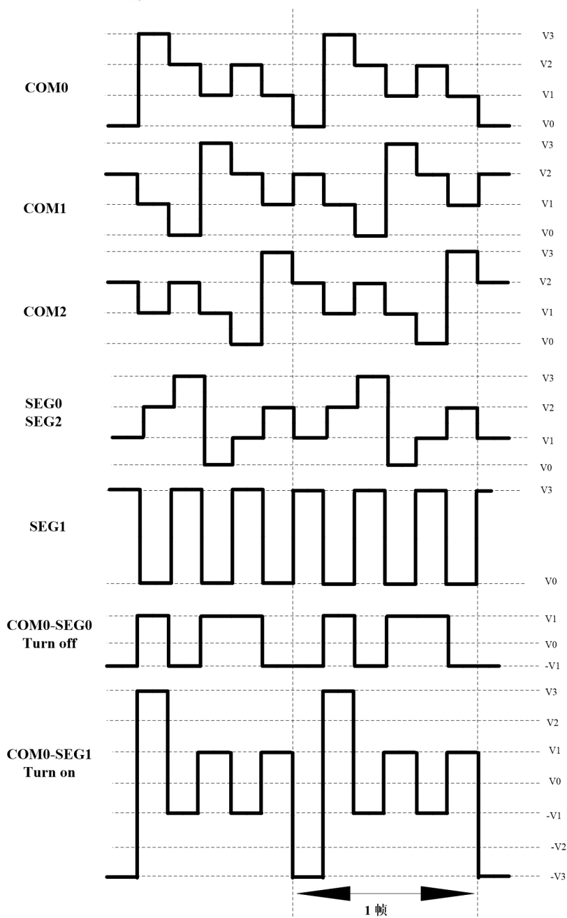
图 16.11 在 1/3 复用、1/3 偏置驱动时的 A 型波形
