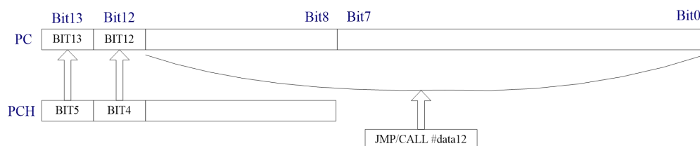
图 3.5 执行 JMP/CALL 指令时 PC 的变化图
