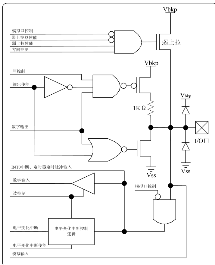
图 2.3.2 P0.3-P0.6 口引脚原理框图
