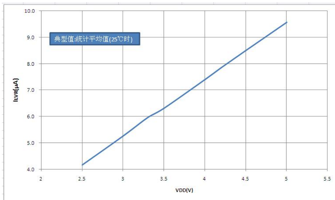
图 25.10:欠压复位电流 I_{LVR} — V_{DD} 关系曲线图
