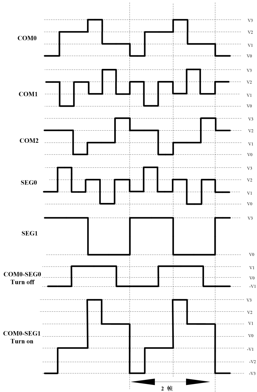
图 16.12 在 1/3 复用、1/3 偏置驱动时的 B 型波形
