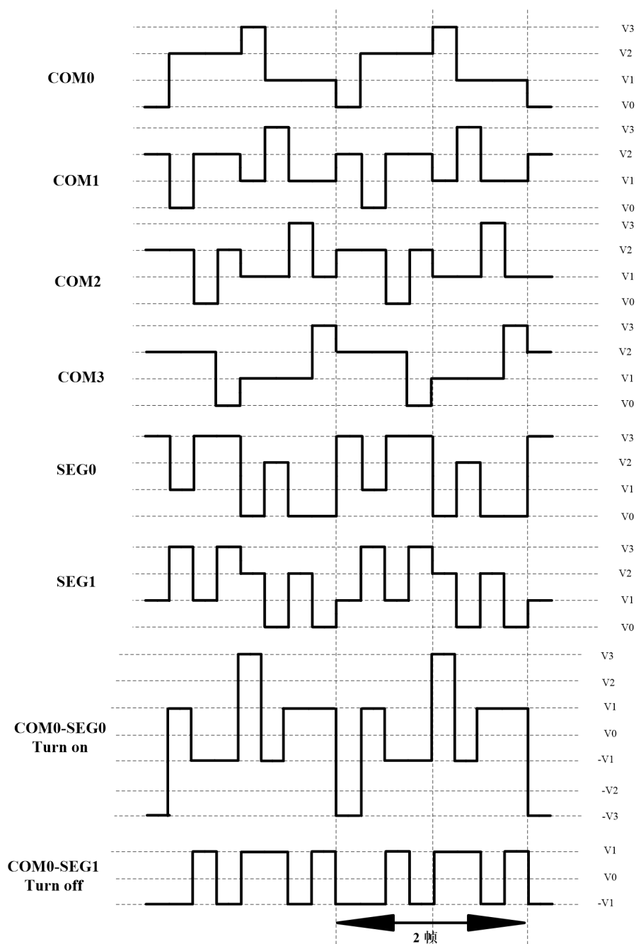
图 16.14 在 1/4 复用、1/3 偏置驱动时的 B 型波形
