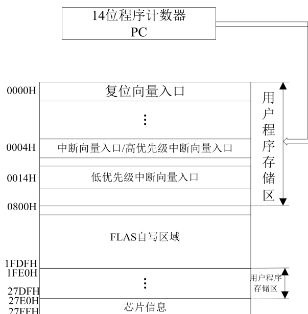
图 3.2 KF8L22Z20XX 程序存储器映射
