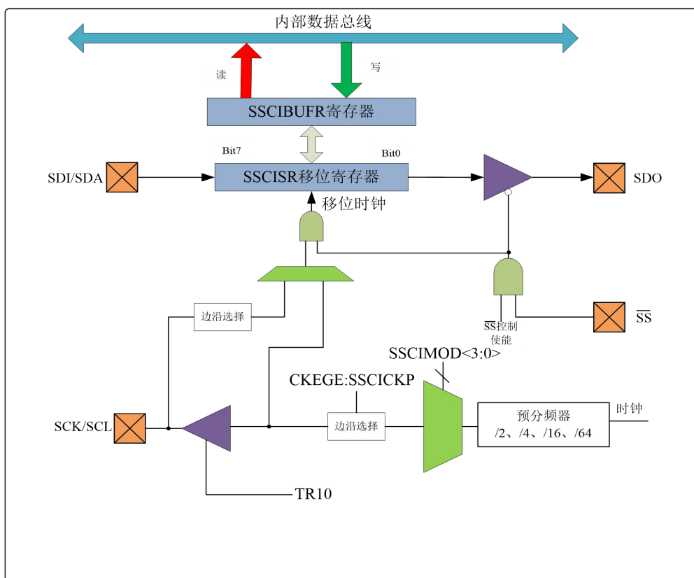
图 13.28 SPI 原理框图
