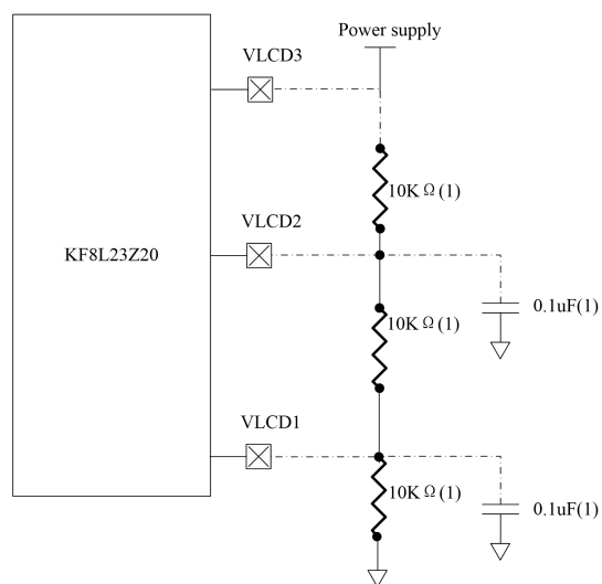
图 16.5 LCD 使用外部分压电阻串时外围推荐线路
