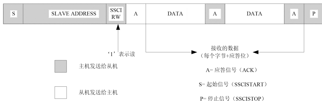
图13.15 I2C协议典型读数据帧格式
