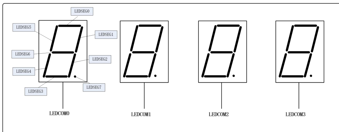
图 15.2 LED 驱动模块与数码管连接示意图
