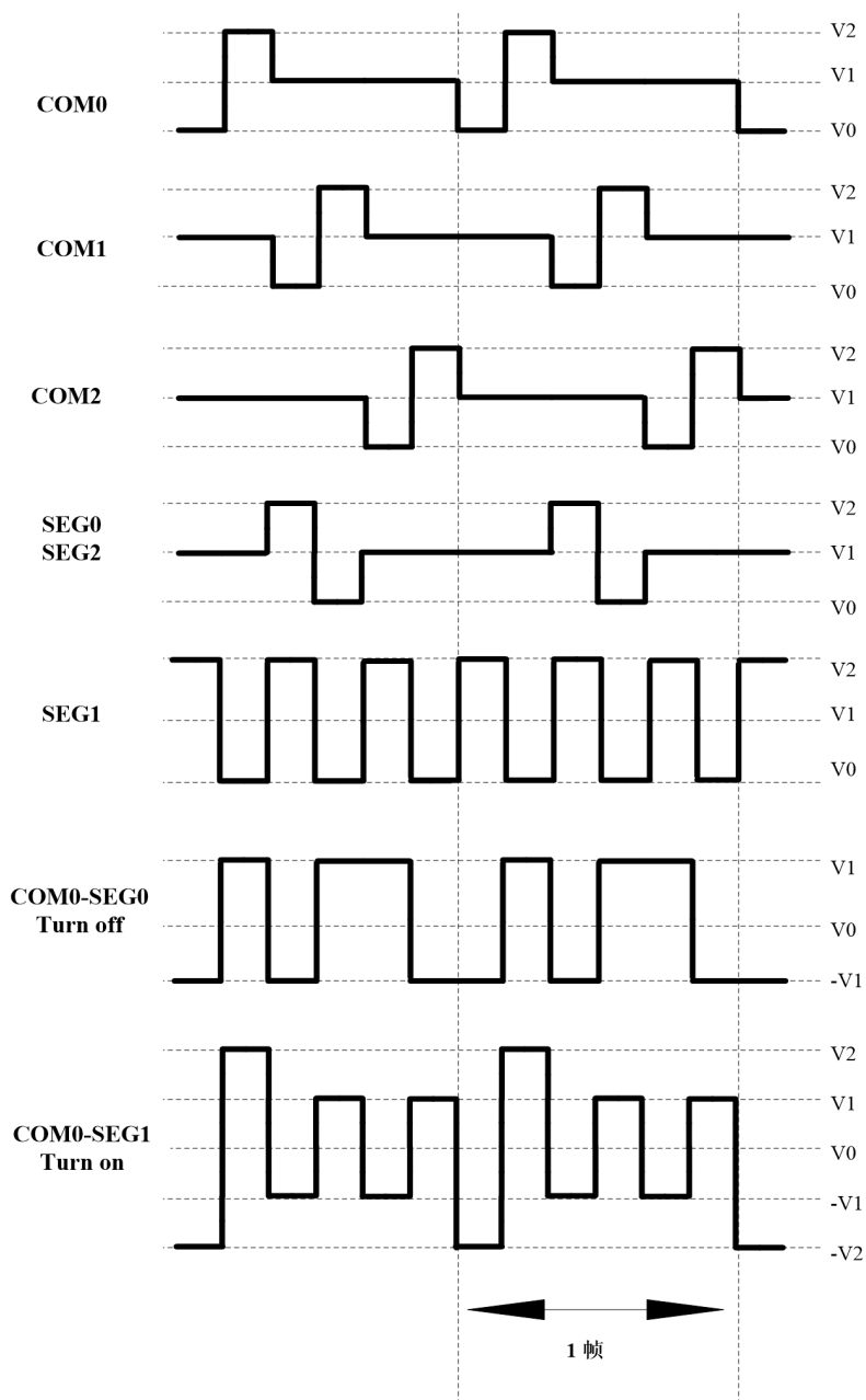
图 16.9 在 1/3 复用, 1/2 偏置驱动时的 A 型波形
