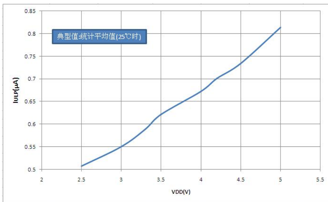
图25.4: 不同VDD 时典型IULP — VDD 关系曲线图(超低功耗模式, 禁止所有外设)
