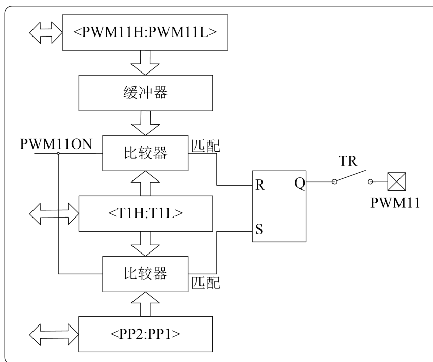
图 9.1 PWM11 逻辑框图
