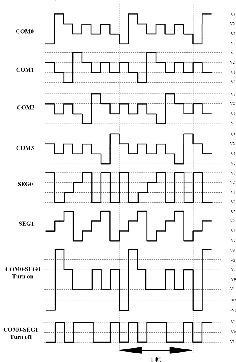
图 16.13 在 1/4 复用、1/3 偏置驱动时的 A 型波形
