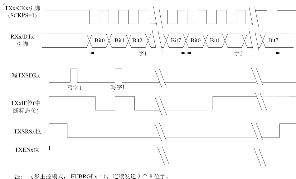
图 14.13 半双工同步发送(SCKPSx=1)
