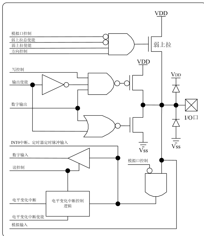
图 2.3.1 P0.0~P0.2、P0.7 口引脚原理框图
