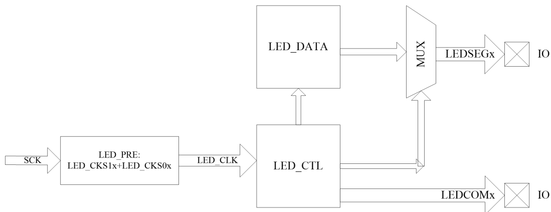
图 15.1 LED 驱动模块框图
