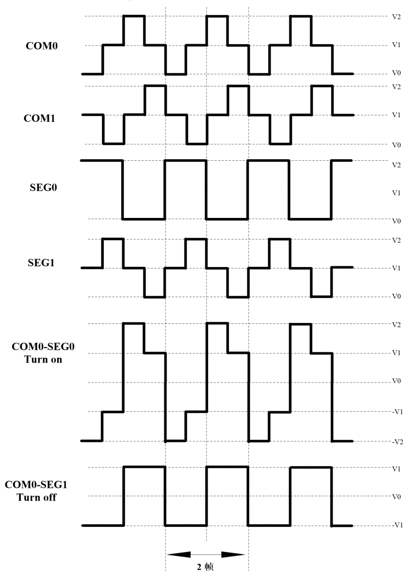
图 16.6 在 1/2 复用、1/2 偏置驱动时的 B 型波形
