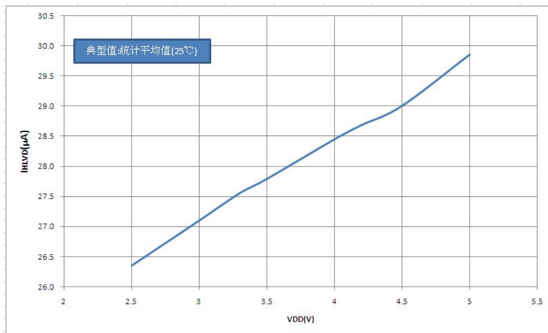
图 25.11: 欠压复位电流 I_{HLVD} — V_{DD} 关系曲线图
