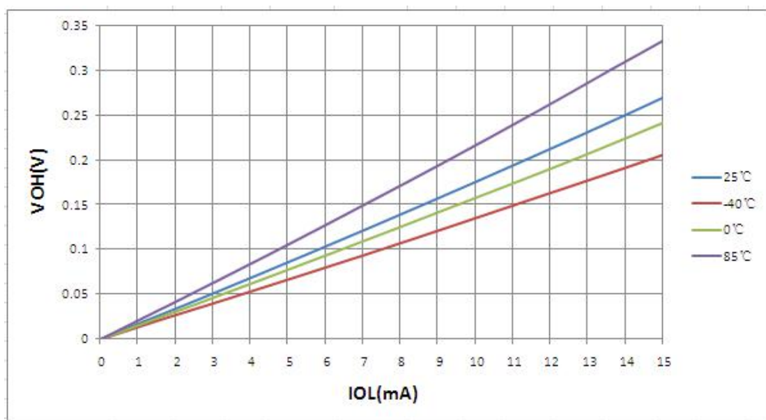
图25.18:不同温度时 V_{OH} — I_{OL} 关系曲线图 ( V_{DD} = 3.0V )
