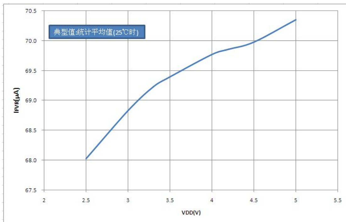
图 25.14: 欠压复位电流 I_{FVR} — V_{DD} 关系曲线图
