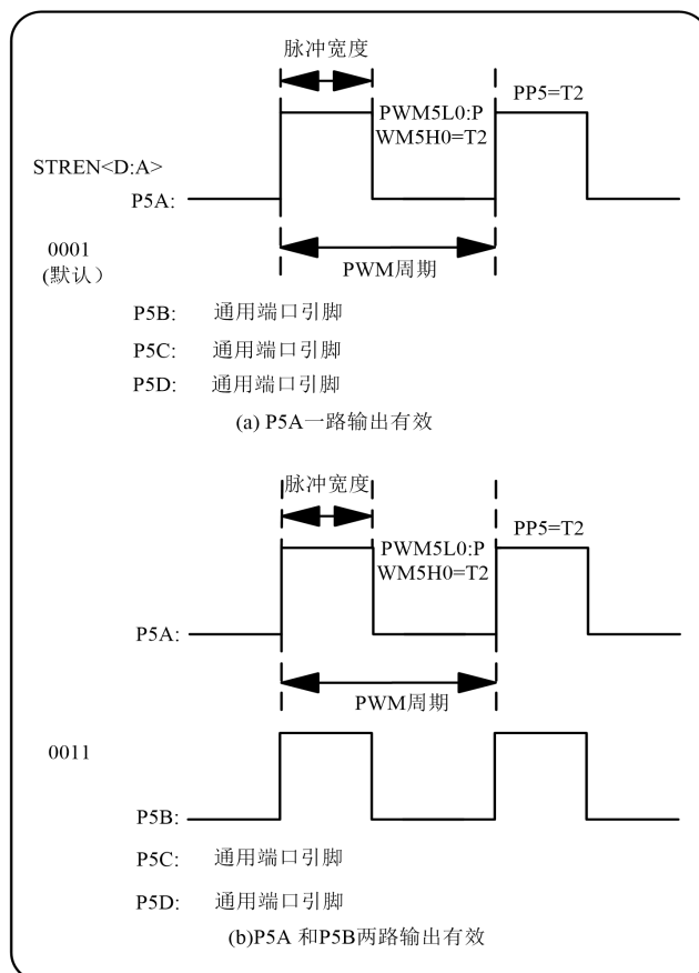
图 10.6 PWM5 的输出示例
