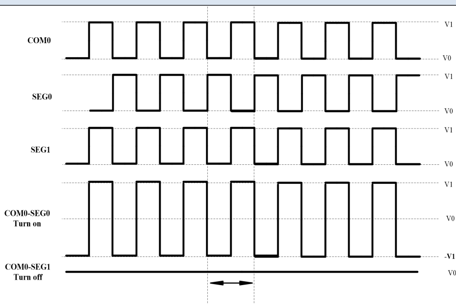
图 16.4 在静态驱动时 A/B 型波形
