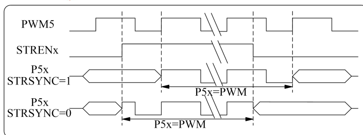
图 10.7 单输出模式 PWM 输出引脚切换
