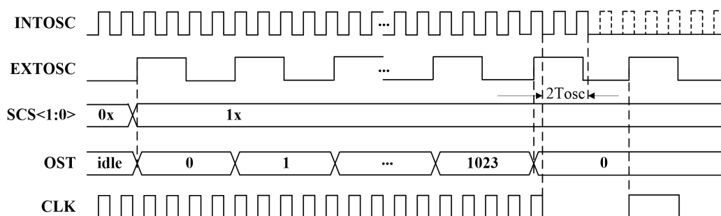
图 1.7 切换至外部时钟源时时钟信号同步时序图
