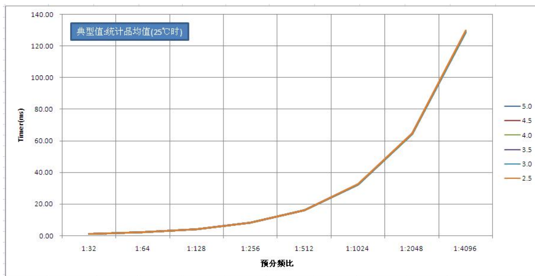
图25.6: 不同VDD时看门狗预分频比PS<2:0> 一周关系曲线图
