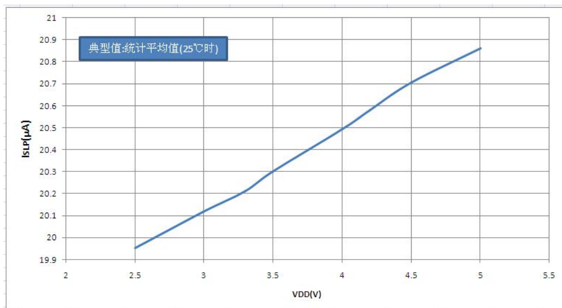
图25.2: 不同VDD 时典型ISLP — VDD 关系曲线图(普通休眠模式, 禁止所有外设)
