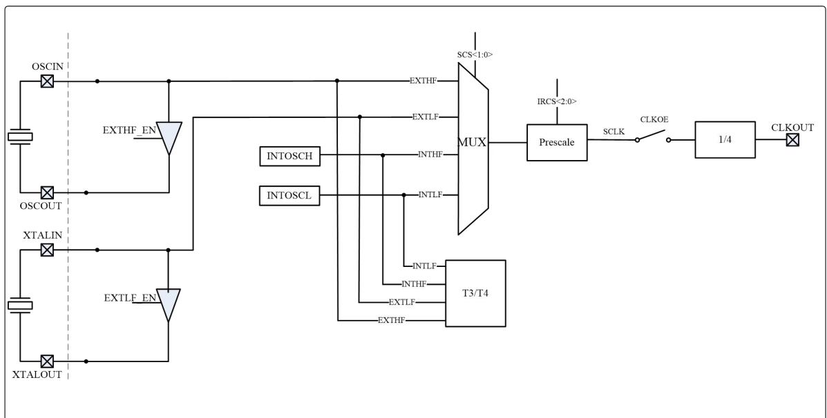
图 1.2 时钟模块原理框图
