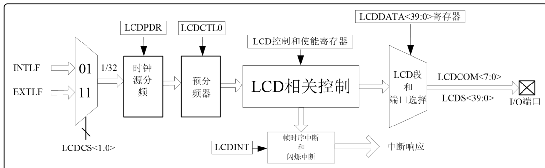
图 16.1 LCD 显示框图
