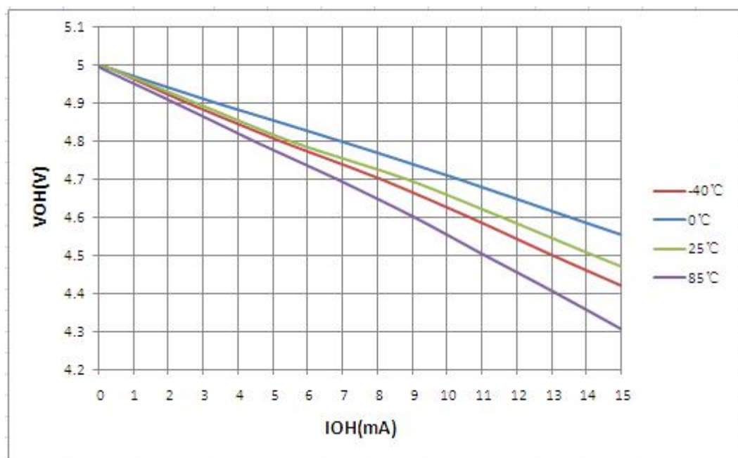
图25.15:不同温度时 V_{OH} — I_{OH} 关系曲线图 ( V_{DD} = 5.0V )
