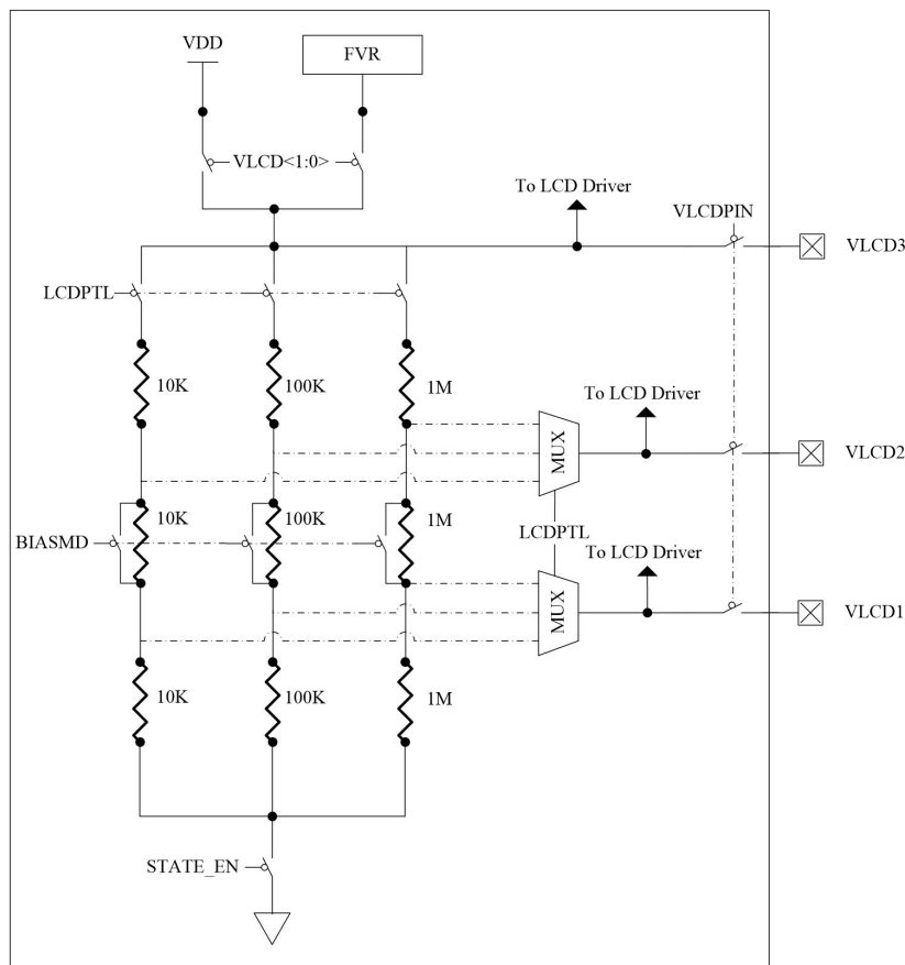
图 16.3 LCD 偏置电路原理框图
