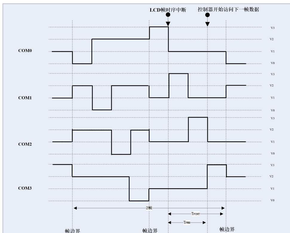
图 16.15 帧时序中断例图
