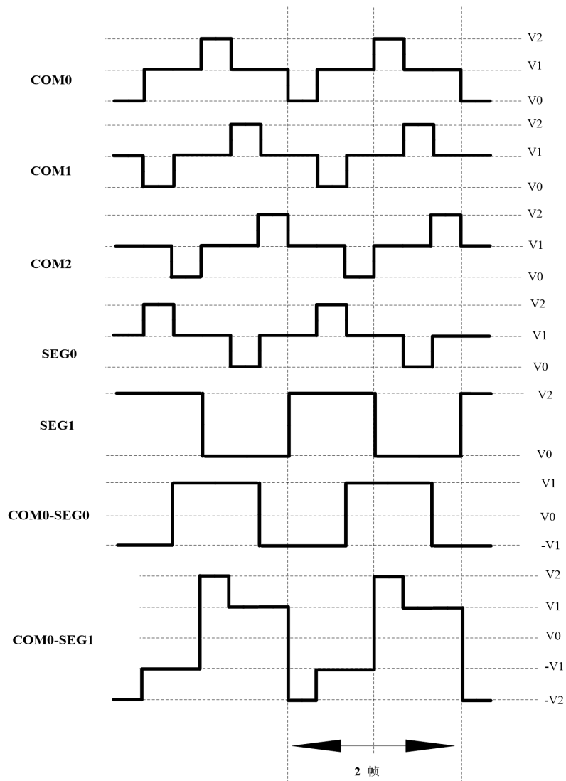
图 16.10 在 1/3 复用、1/2 偏置驱动时的 B 型波形
