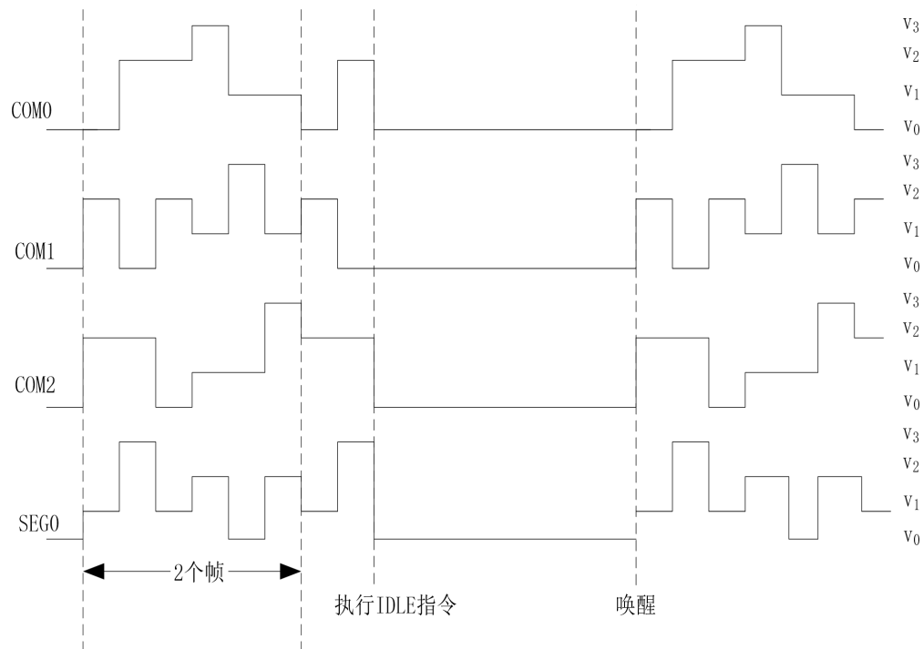
图 16.16 当 \overline{\text{SLPEN}} = 1 是进入/退出休眠模式
