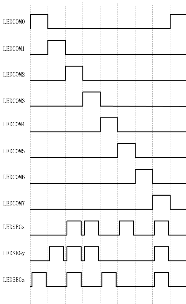
图 15.3 LED 扫描波形例图(使能 8 位)
