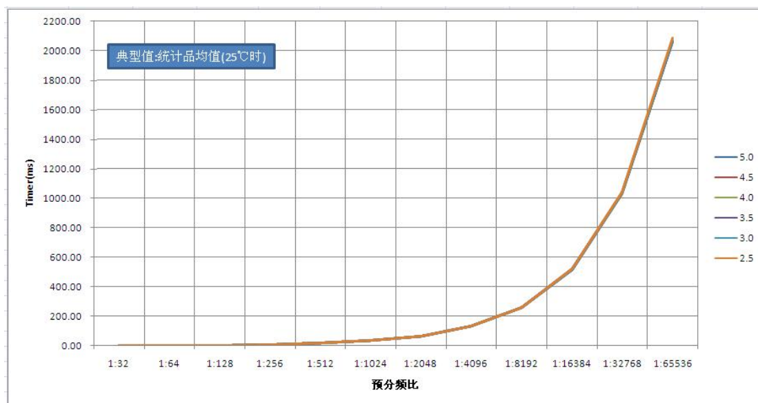
图25.5: 不同VDD时看门狗预分频比WDTPS<3:0> 一周关系曲线图
