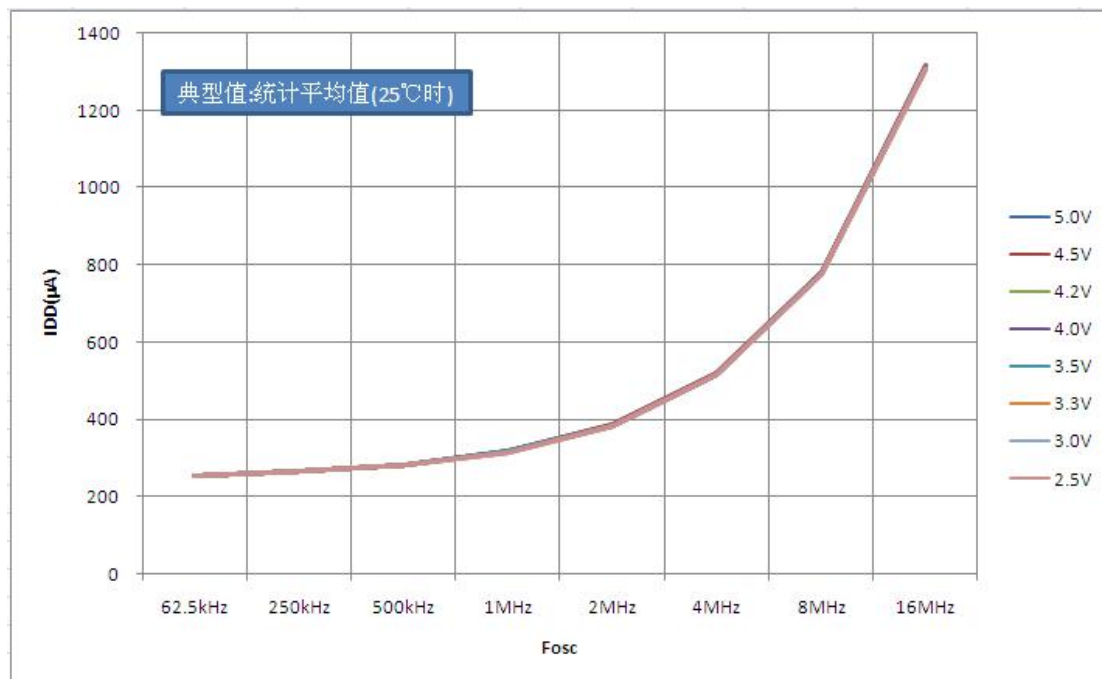
图25.1: 不同VDD 时典型IDD — FOSC 关系曲线图(HFINTOSC模式)
