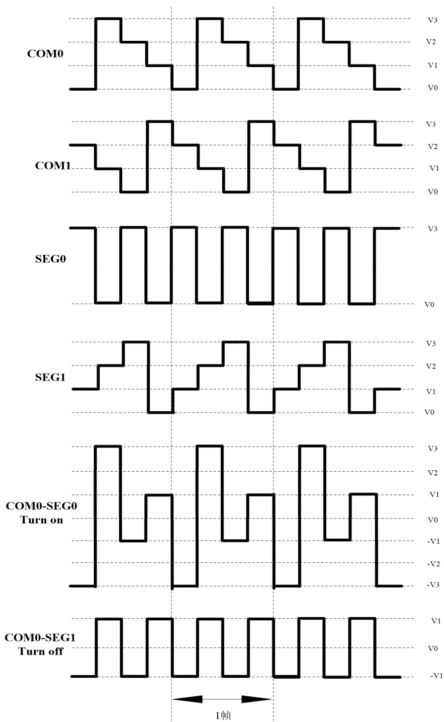
图 16.7 在 1/2 复用, 1/3 偏置驱动时的 A 型波形
