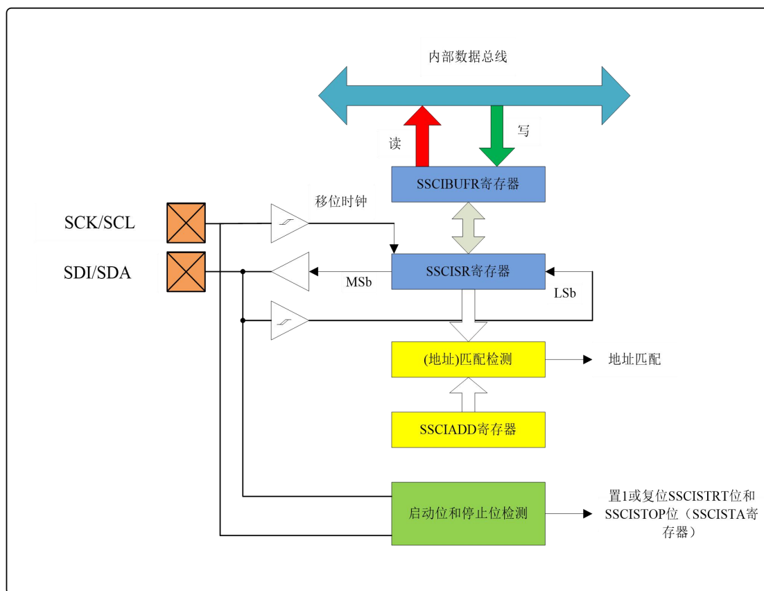
图13.1 I2C模式方框图
