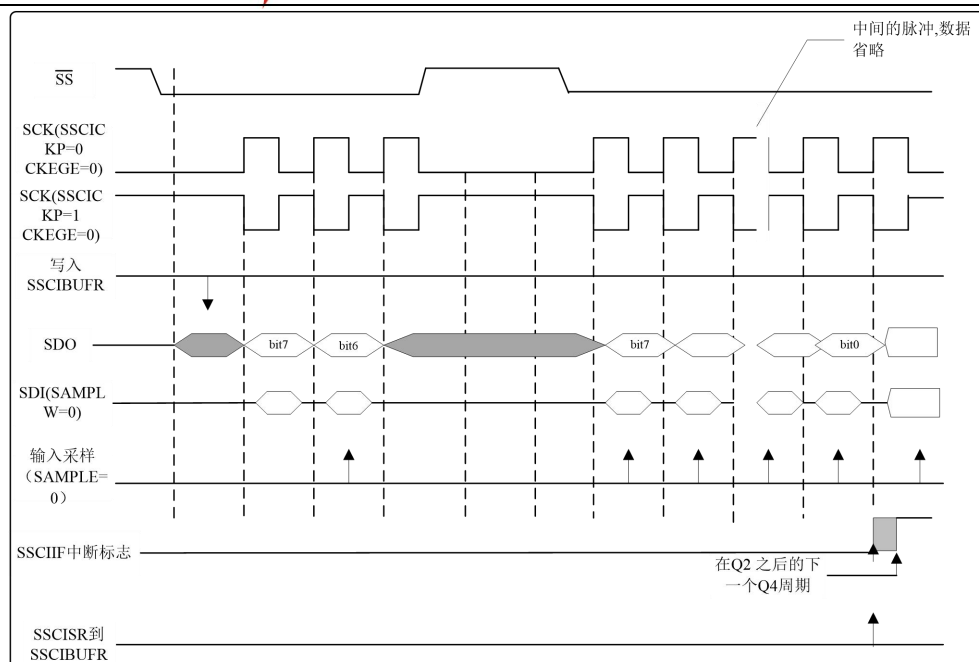
图13.31 从动时序图
