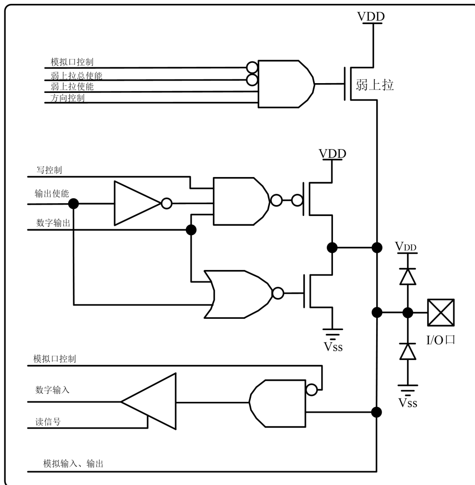
图 2.10 P7 口引脚原理功能框图
