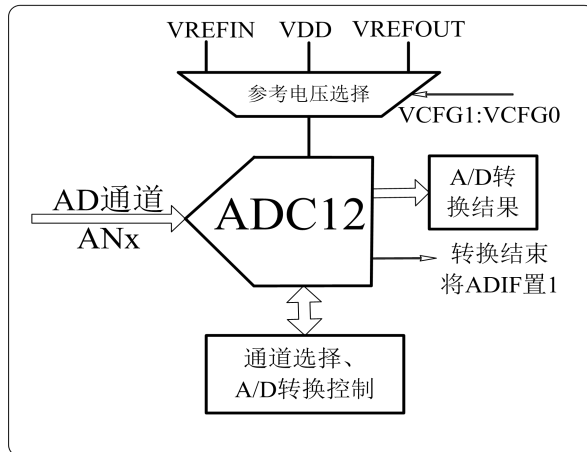
图 7.1 ADC12 模块结构框图
