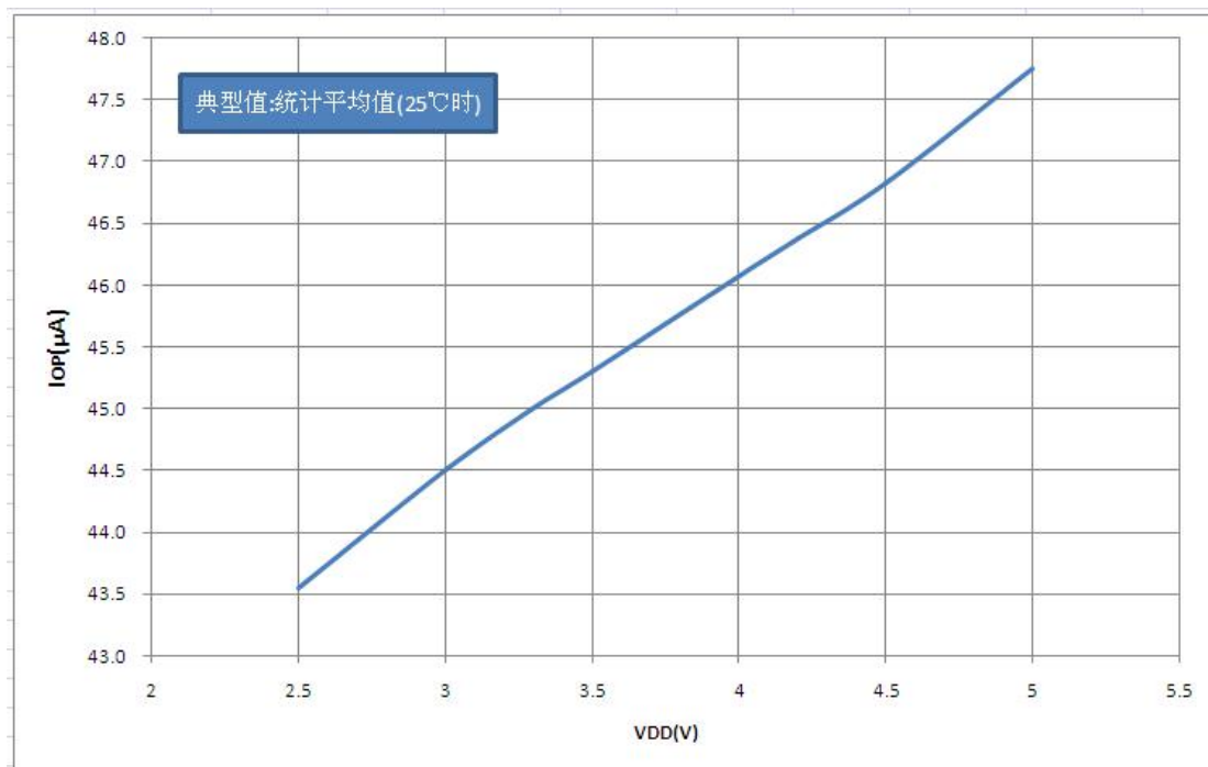
图25.9:运算放大器电流 I_{OP} — V_{DD} 关系曲线图（使能一路比较器）
