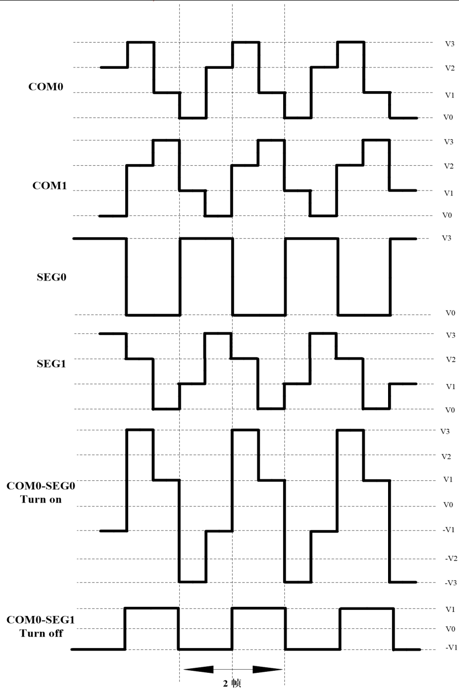
图 16.8 在 1/2 复用、1/3 偏置驱动时的 B 型波形
