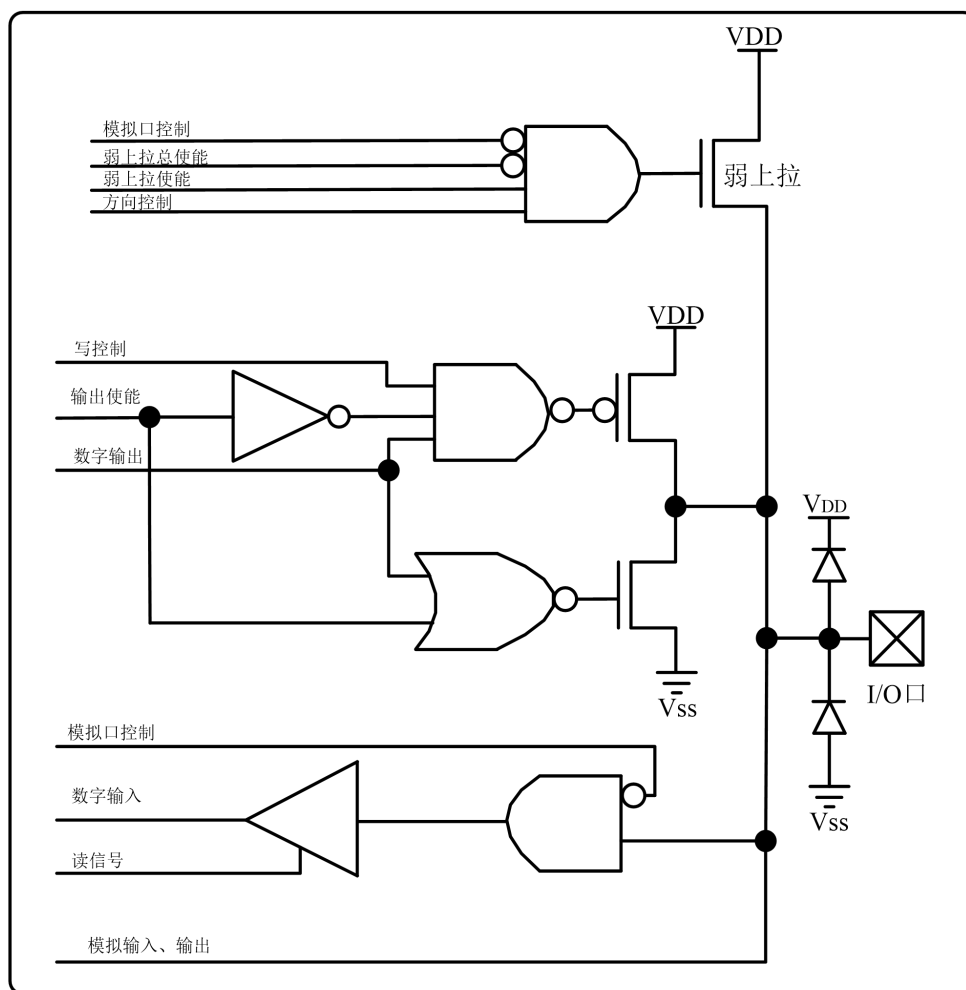
图 2.9 P6 口引脚原理功能框图
