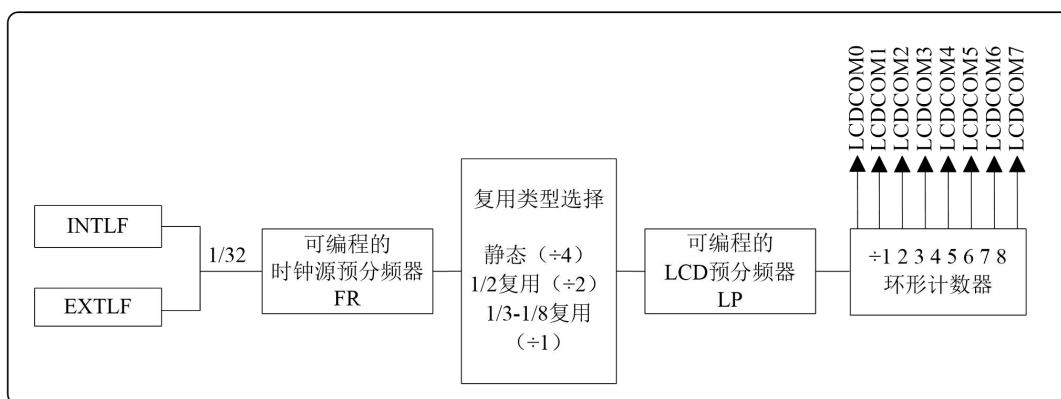
图 16.2 LCD 预分频器图
