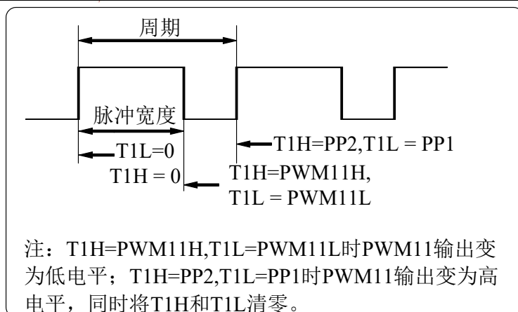
图 9.2 PWM11 输出波形图
