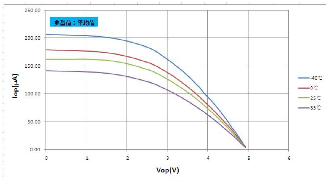
图25.19:上拉功能打开时端口电压VOP — 电流IOP 关系曲线图 (VDD = 5.0V)
