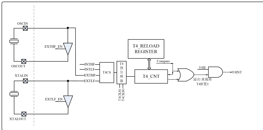
图 6.7 T4 原理框图
