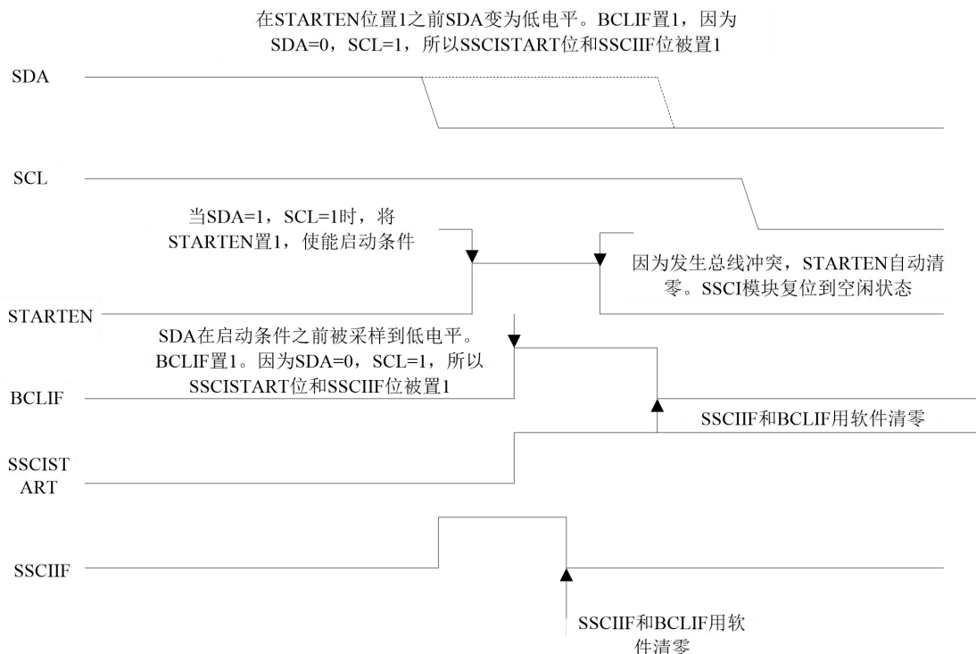
图13.21 启动条件期间的总线冲突（仅SDA）
