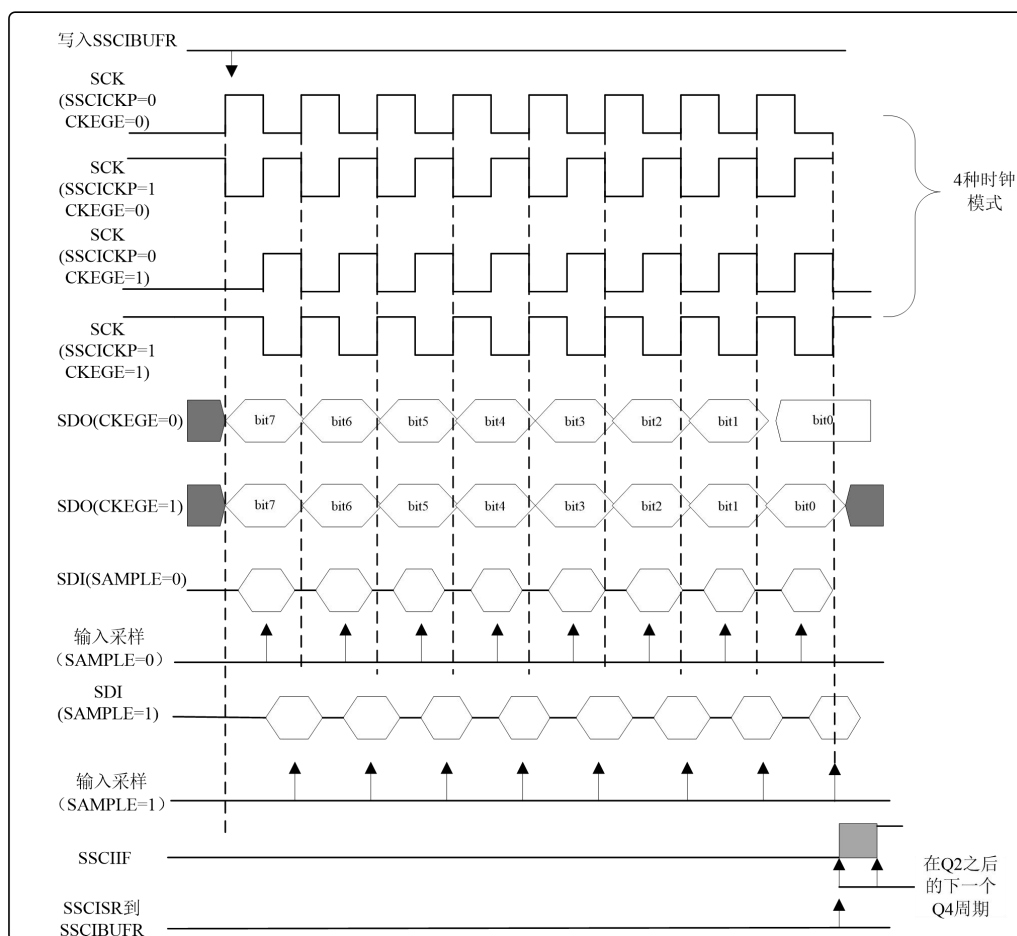
图 13.30 SPI 主控模式时序图
