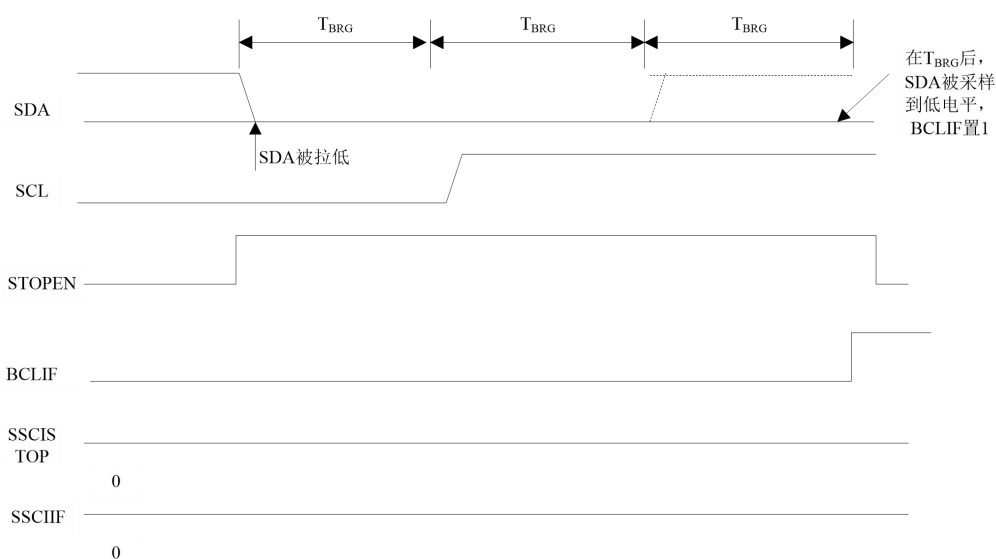
图13.26 停止条件期间的总线冲突(情形1)
