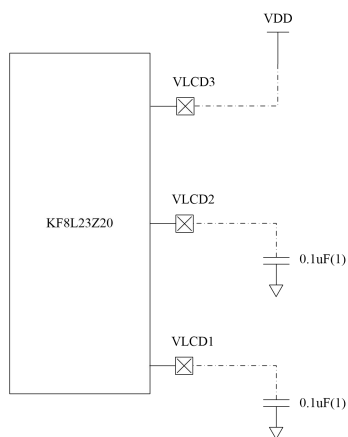
图 16.4 LCD 使用内部分压电阻串时外围推荐线路
