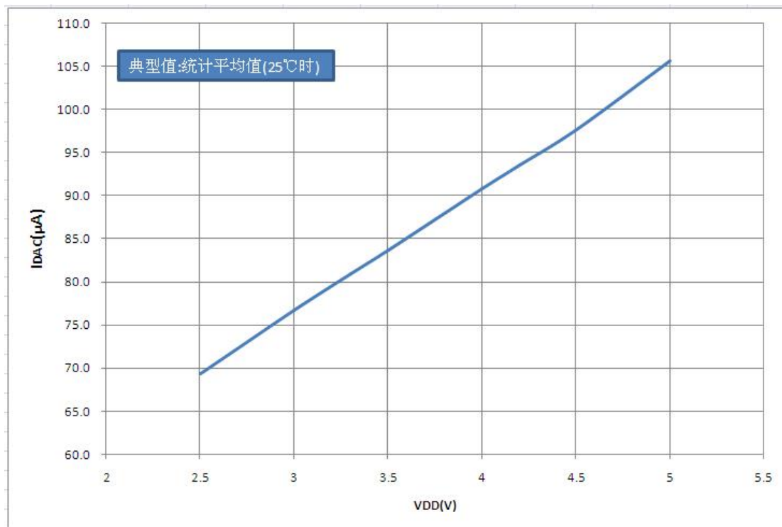
图 25.13: 欠压复位电流 I_{DAC} — V_{DD} 关系曲线图
