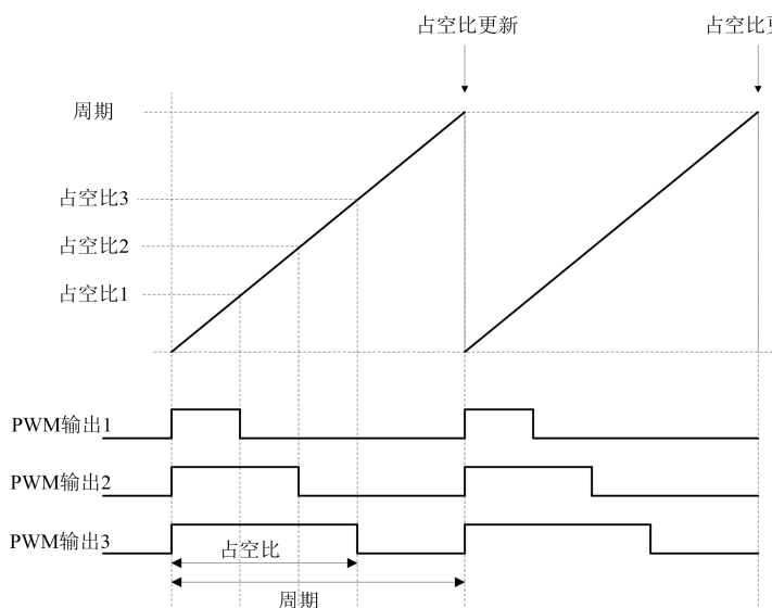
图 10.4 边沿对齐 PWM
