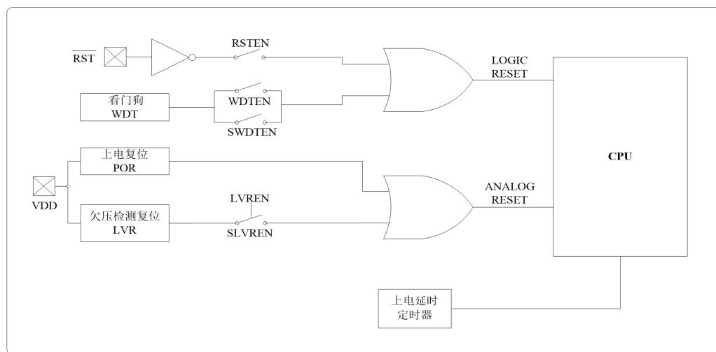
图 22.1 片内复位电路简化框图
