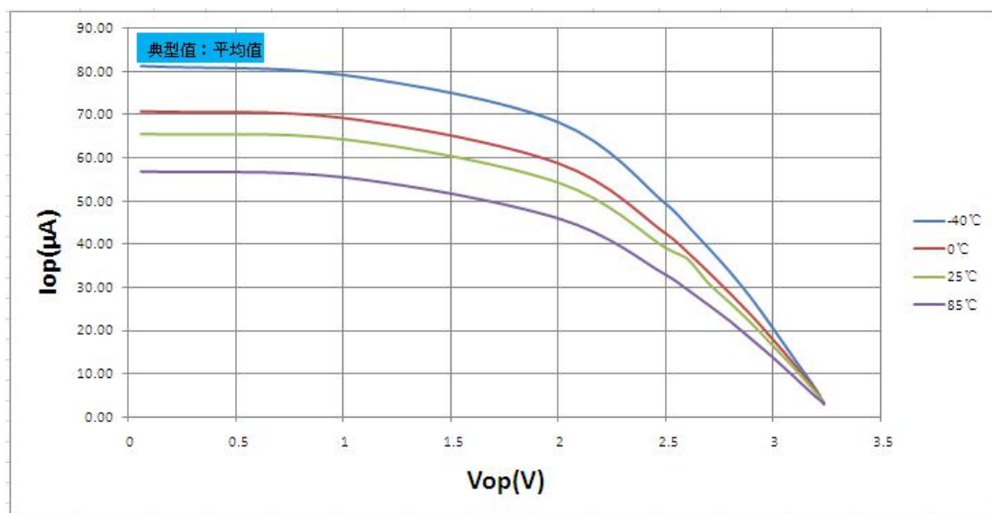
图25.20:上拉功能打开时端口电压VOP — 电流IOP 关系曲线图 (VDD = 3.3V)
