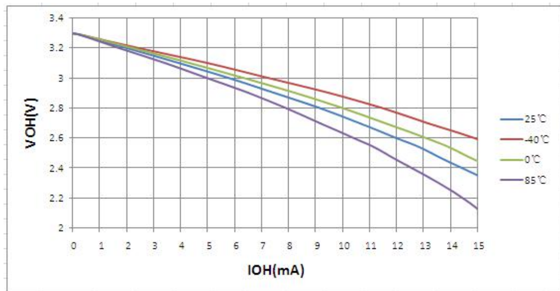
图25.16:不同温度时 V_{OH} — I_{OH} 关系曲线图 ( V_{DD} = 3.0V )
