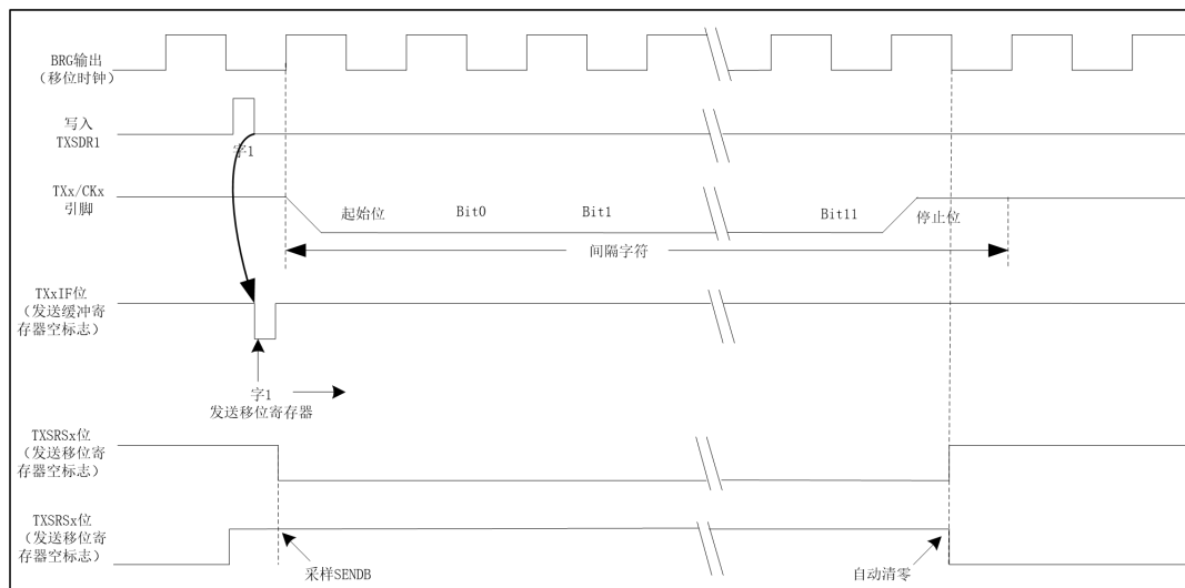
图 14.6 发送间隔字符时序
