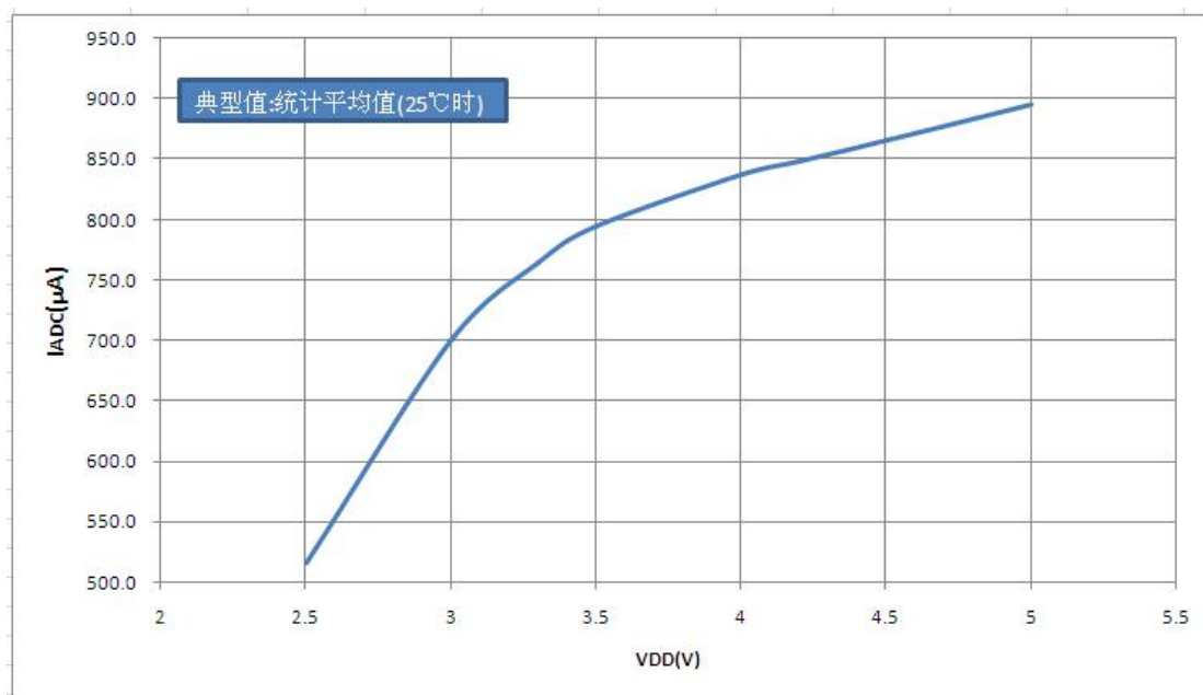
图 25.12: 欠压复位电流 I_{ADC} — V_{DD} 关系曲线图
