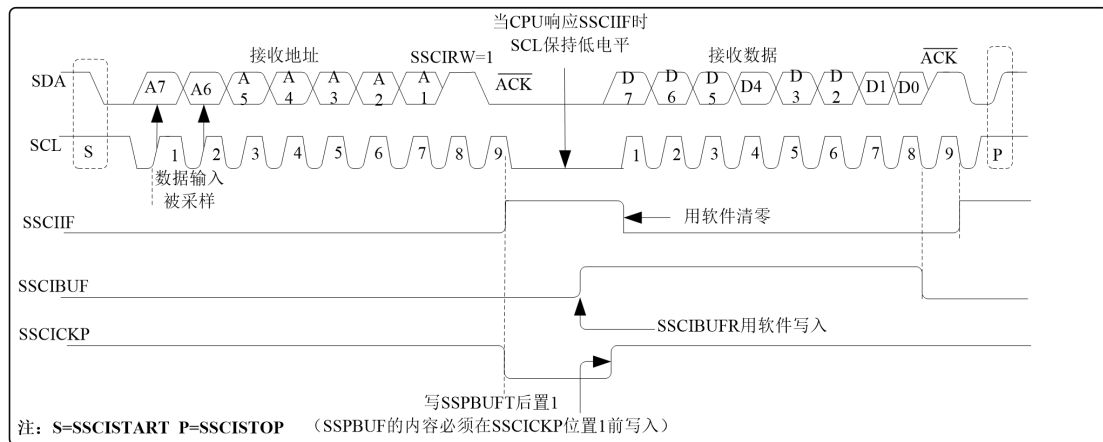
图 13.4 从动模式时序（发送，7 位地址）
