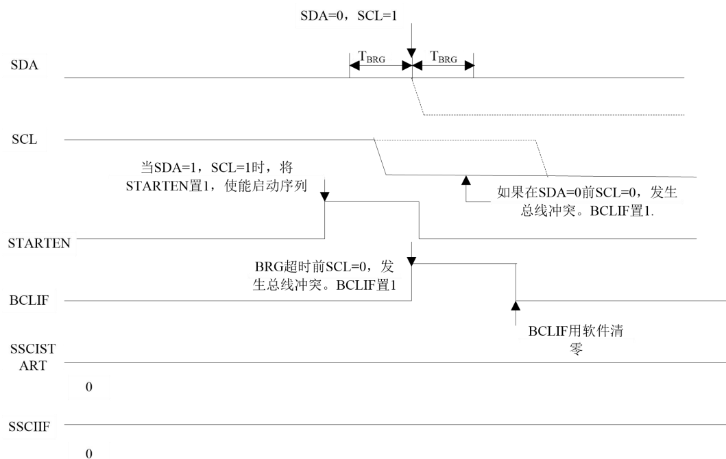
13.22 启动条件期间的总线冲突（SCL=0）
