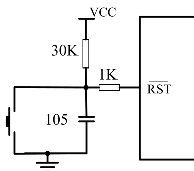
图 22.2 建议 \overline{\text{RST}} 复位电路
