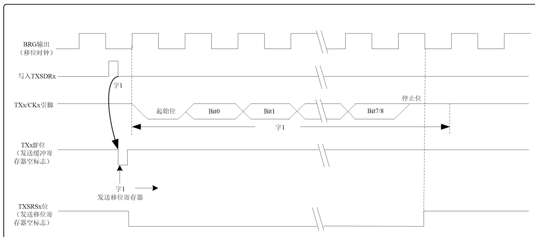
图 14.9 全双工异步发送（两字符间有空闲位）
